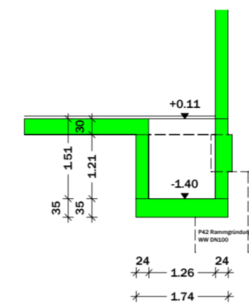
Schnitt P4
