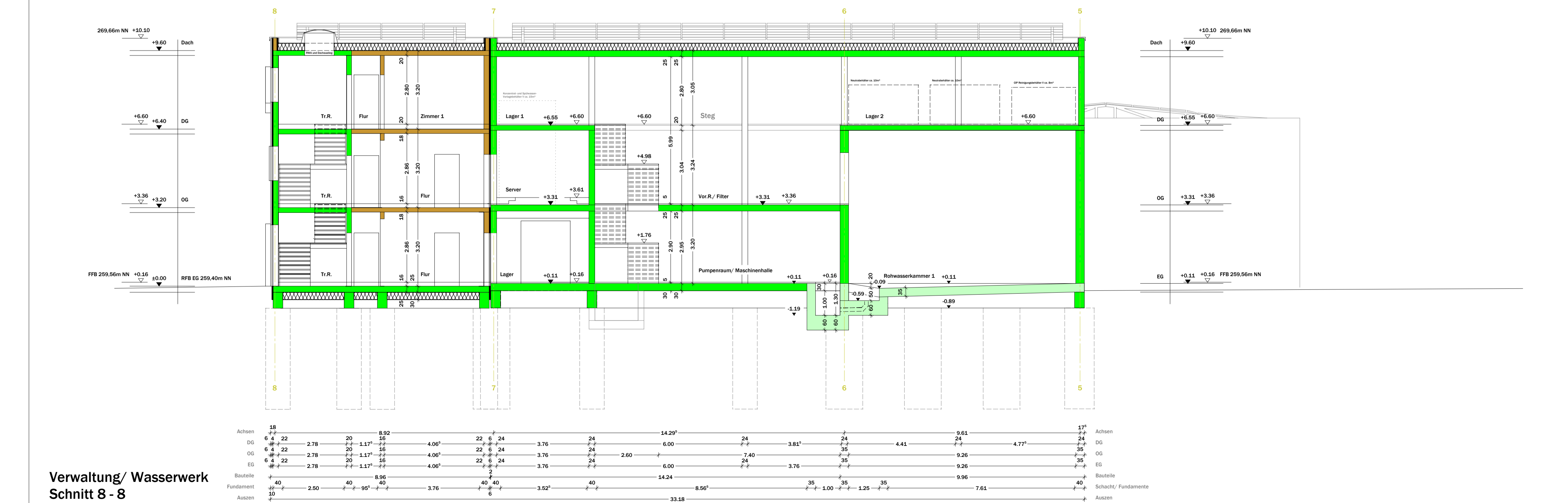
Wasserwerk Schnitt 4 - 4
