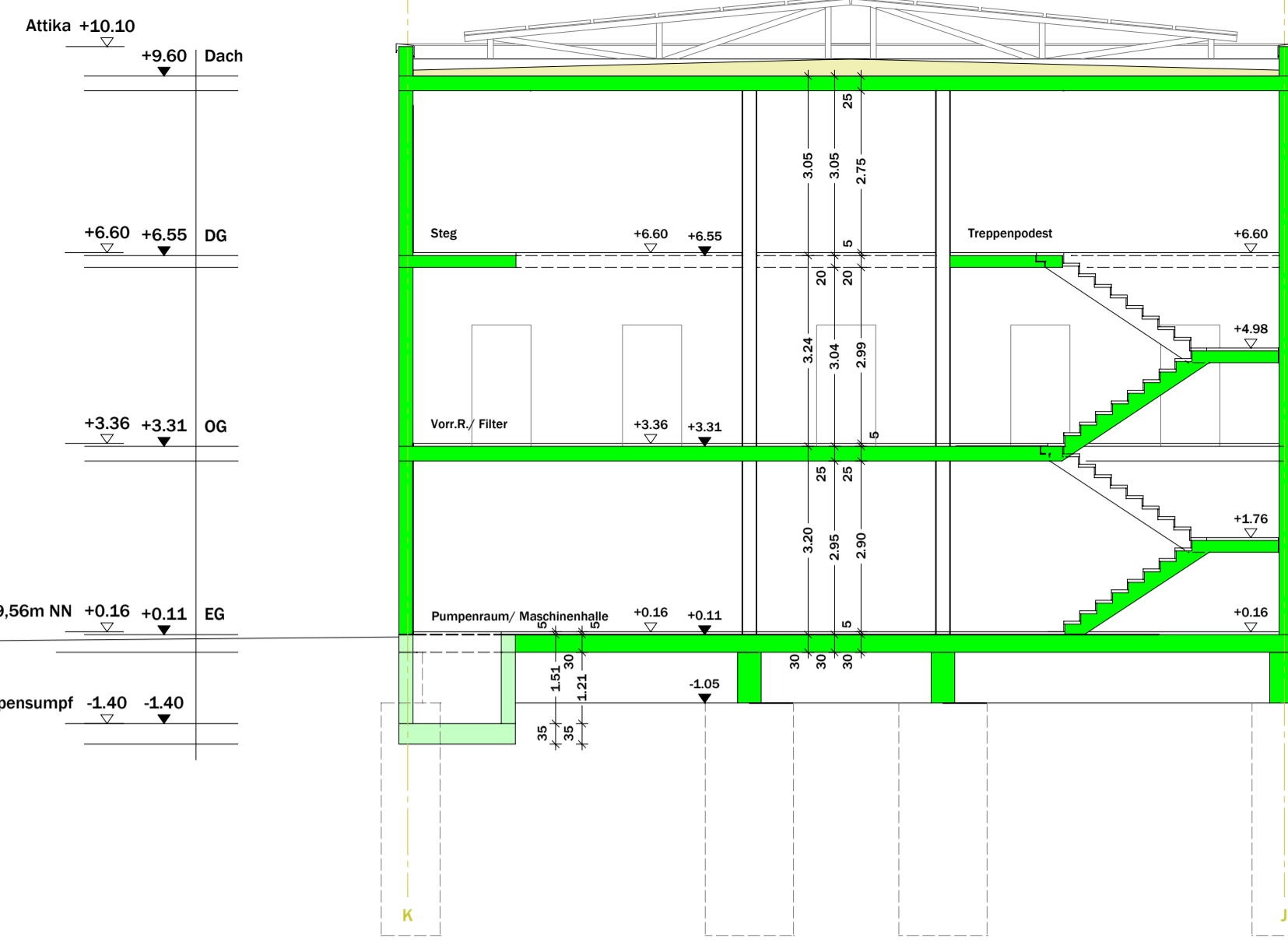
Wasserwerk Schnitt 3 - 3
