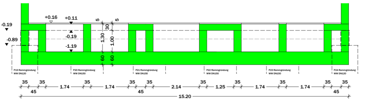
Schnitt P2
