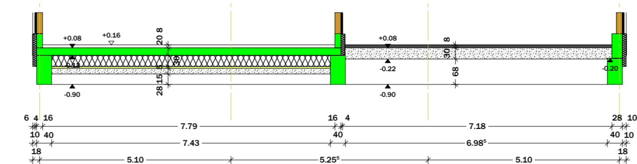
Schnitt P7
