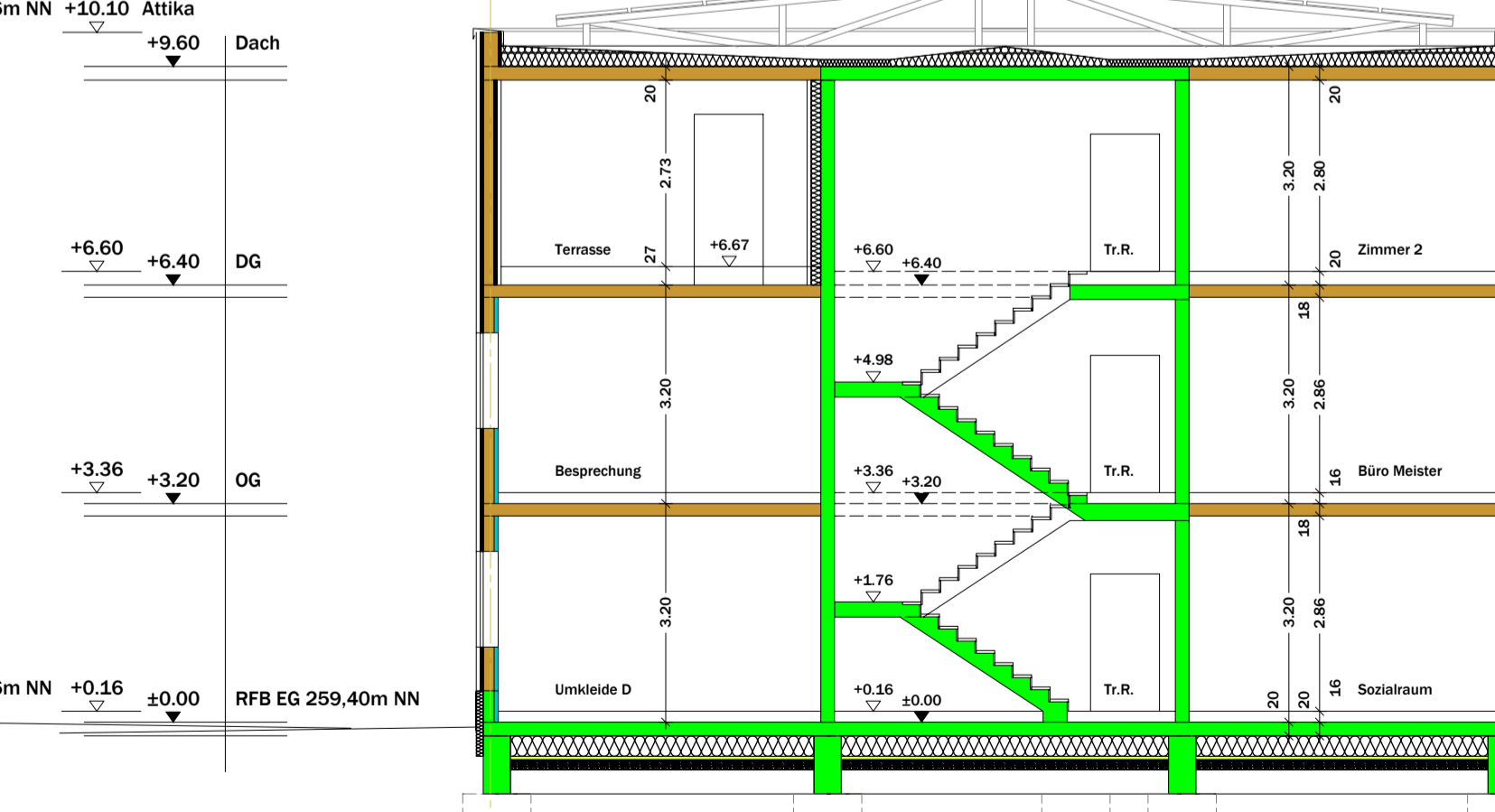
Verwaltung Schnitt 2 - 2
