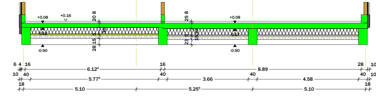
Schnitt P6
