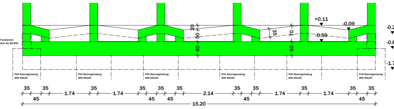
Schnitt P1
