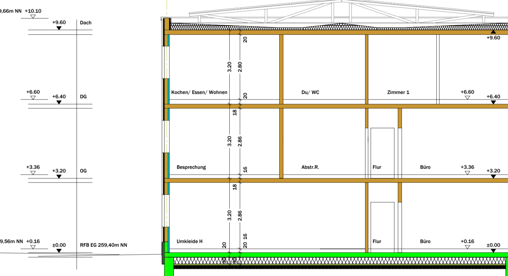
Wasserwerk Schnitt 3 - 3
