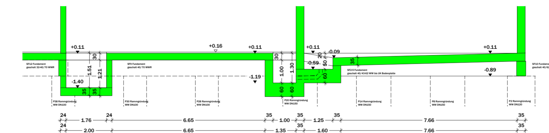
Schnitt P3
